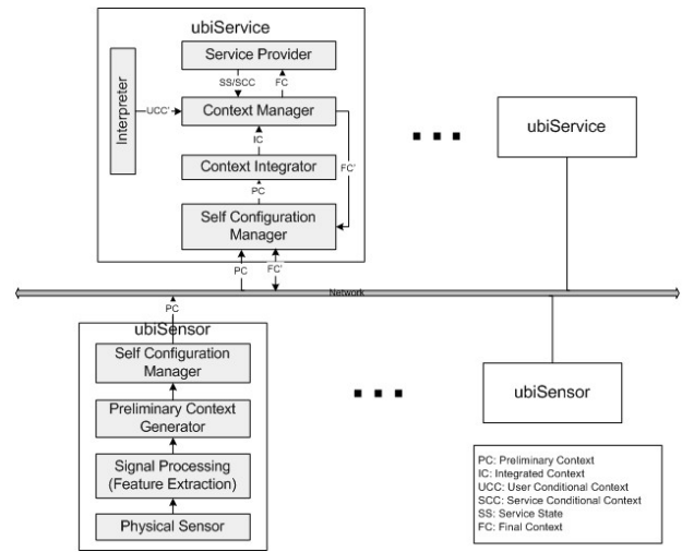
그림 5 ubi-UCAM의 구조
