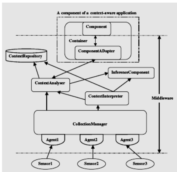
그림 3 CAMidO의 구조
